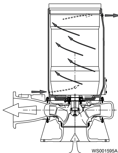
Рис. 8: Пример для пояснения принципа внешнего охлаждения.
