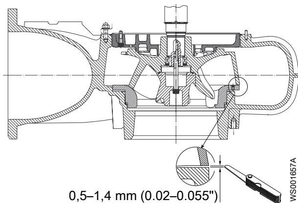
Рис. 100: Измерьте расстояние S
