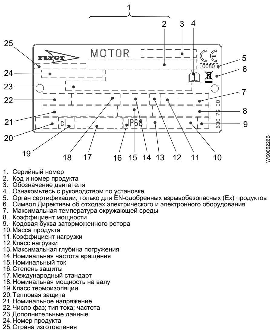
Рис. 11: Табличка для приводного блока начиная с 990101
