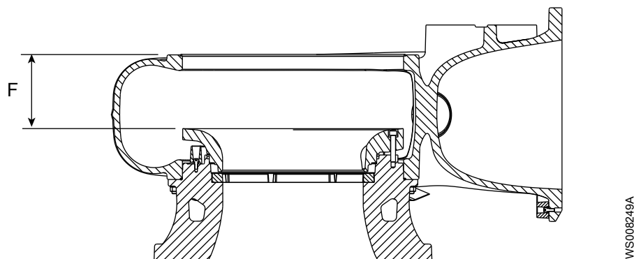
Рис. 96: Измерение расстояния F. Показан стандартный насос N.
