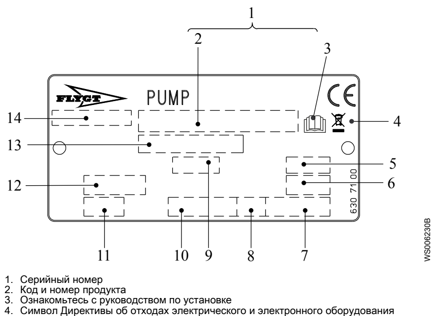
Рис. 11: Табличка для приводного блока начиная с 990101
