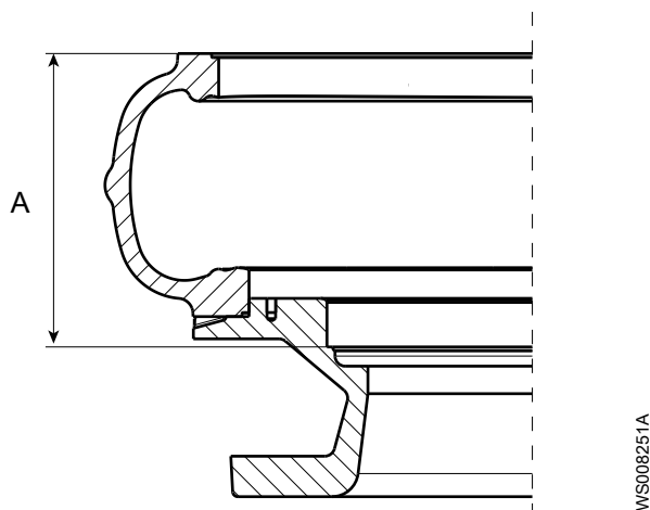
Рис. 97: Измерьте расстояние A
