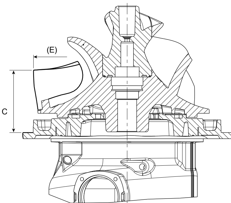
Рис. 95: Измерьте расстояние C.
