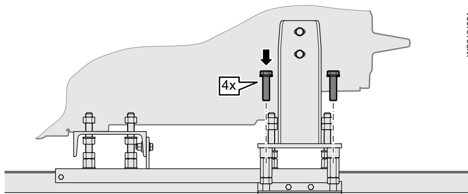
Рис. 91: Вставка болтов внешних опор
